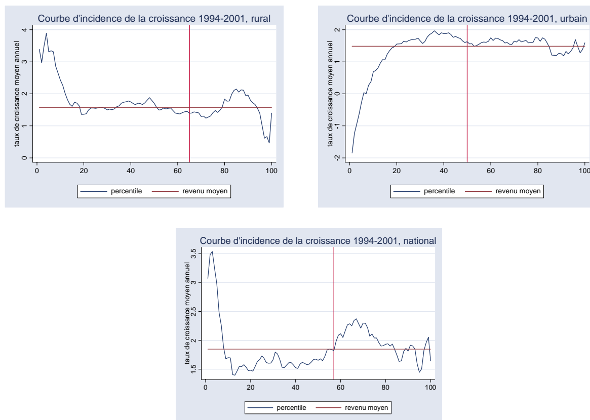
Figure 1 : courbes d'incidence de croissance, niveau national, urbain et rural
